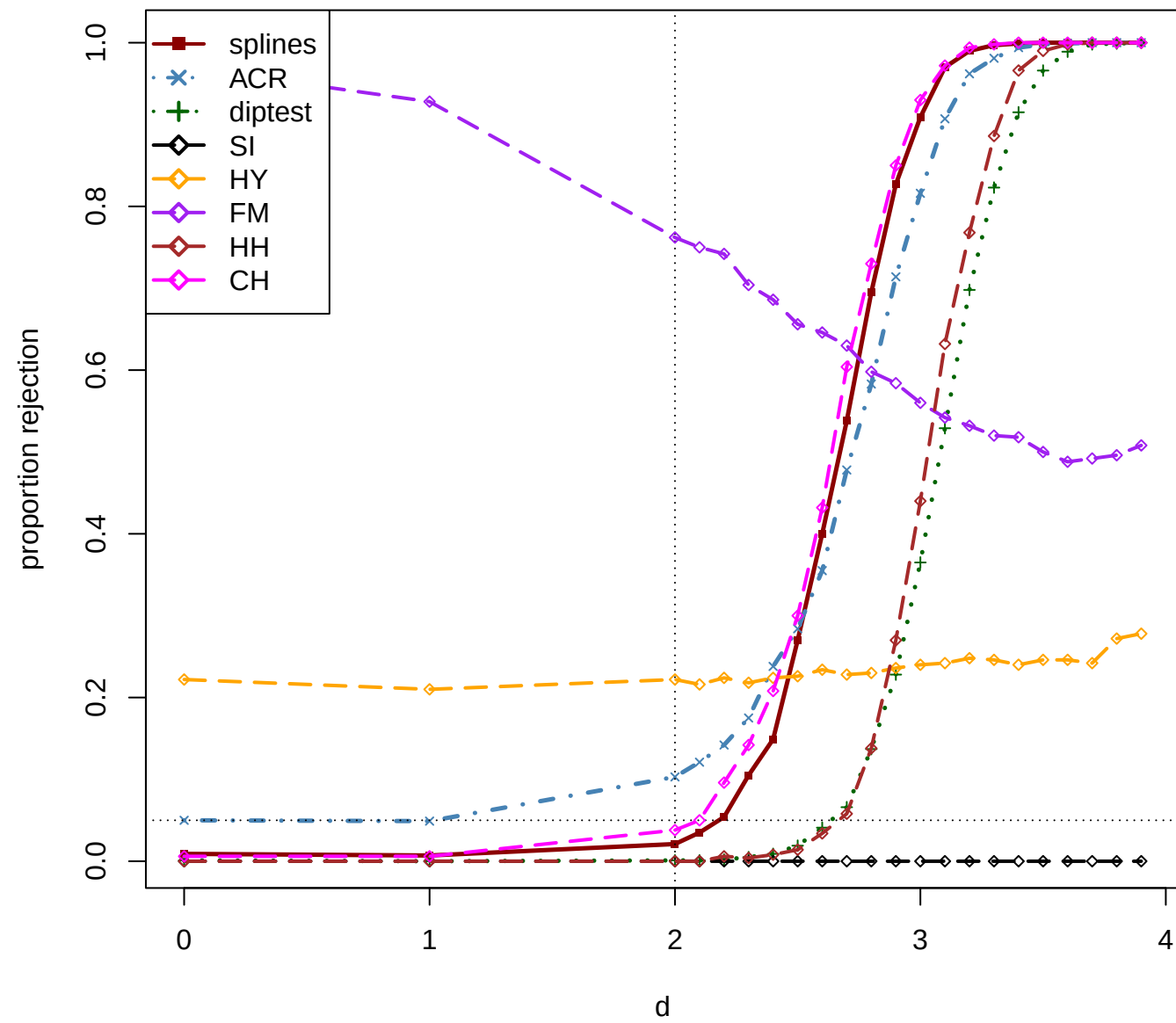
0.4N(0,1)+0.4N(d,1)+0.2N(0,9) , n=800
