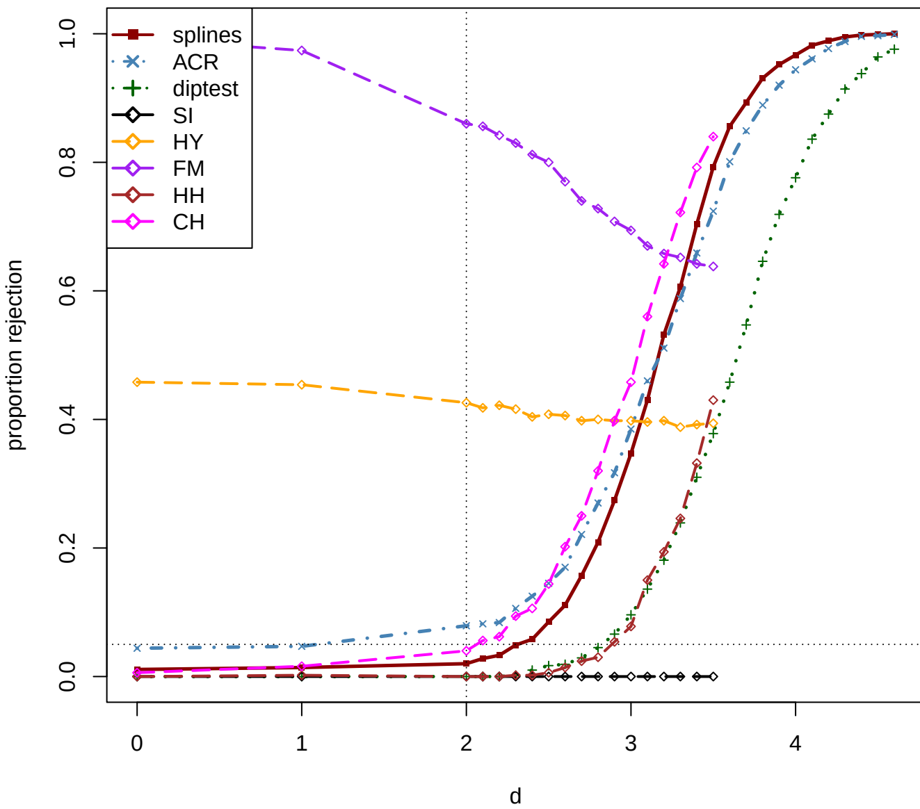
0.4N(0,1)+0.4N(d,1)+0.2N(0,9) , n=200
